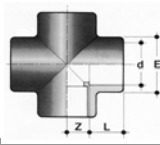
XIV/21.030.01 - Kreuzstück
