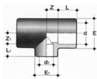
TRIV-переходной тройник
