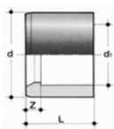
DIV-переходное кольцо
