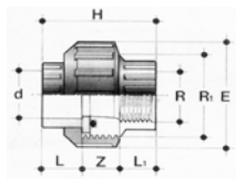
BIFV-разборная муфта с внутр.резьбой, прокладка из ЭПДМ или ФПМ
