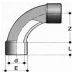
SIV - отвод 90° большого радиуса
