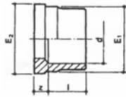
Q/BIV-втулочное окончание для разборной муфты
